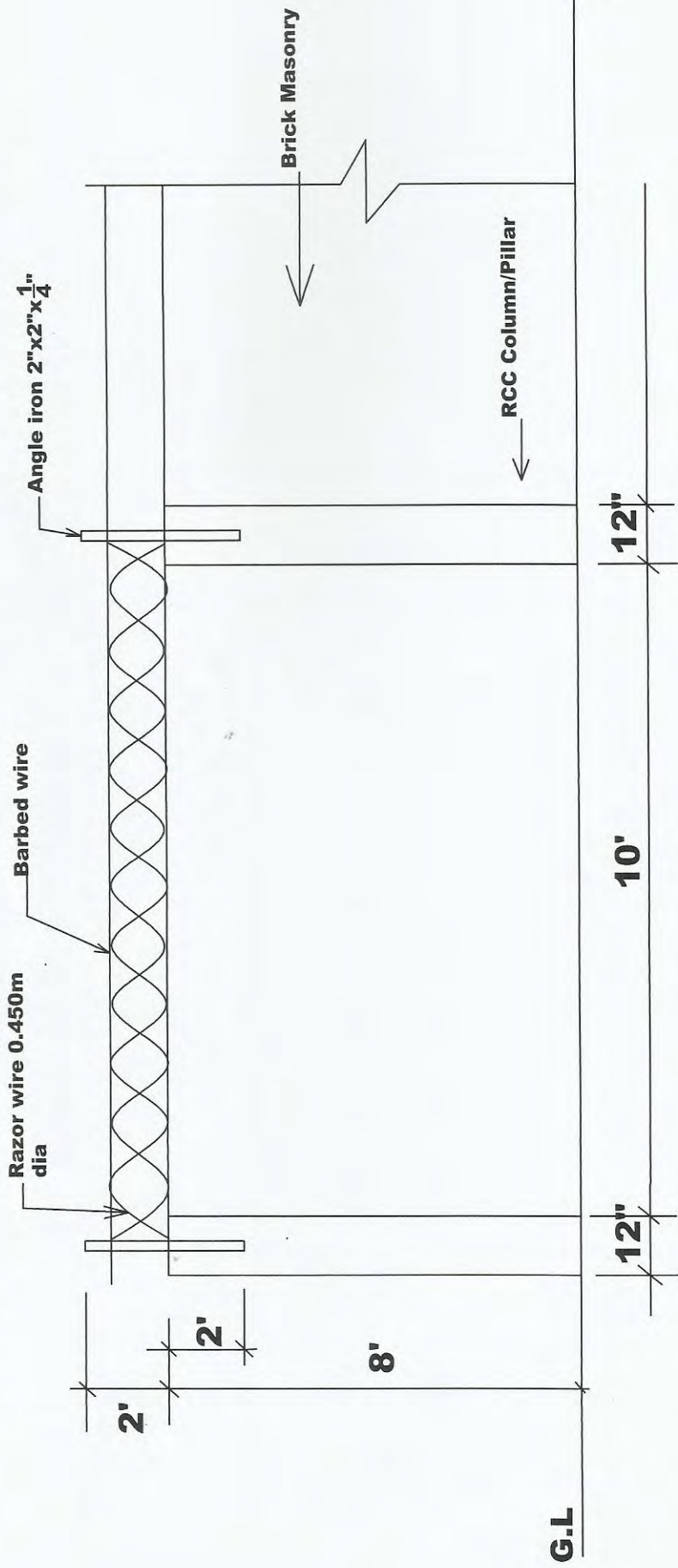
Elevation
