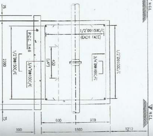
SECTION B-B (SCALE - 1:30)
