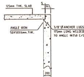
DETAIL-A (SCALE 1:25)
