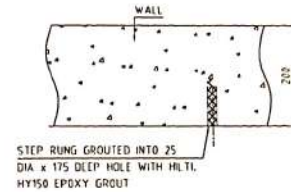
DETAIL-B (SCALE 1:10)
