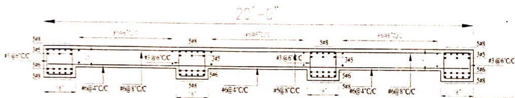
SECTION A-A SCALE: 1/2"=1'-0"
